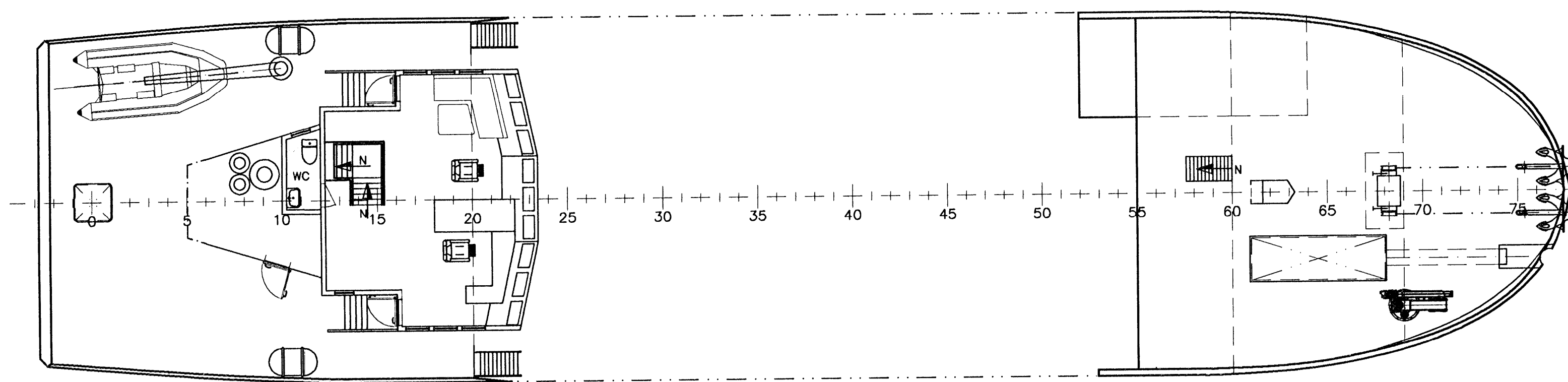
POOP/BAKKDEKK
