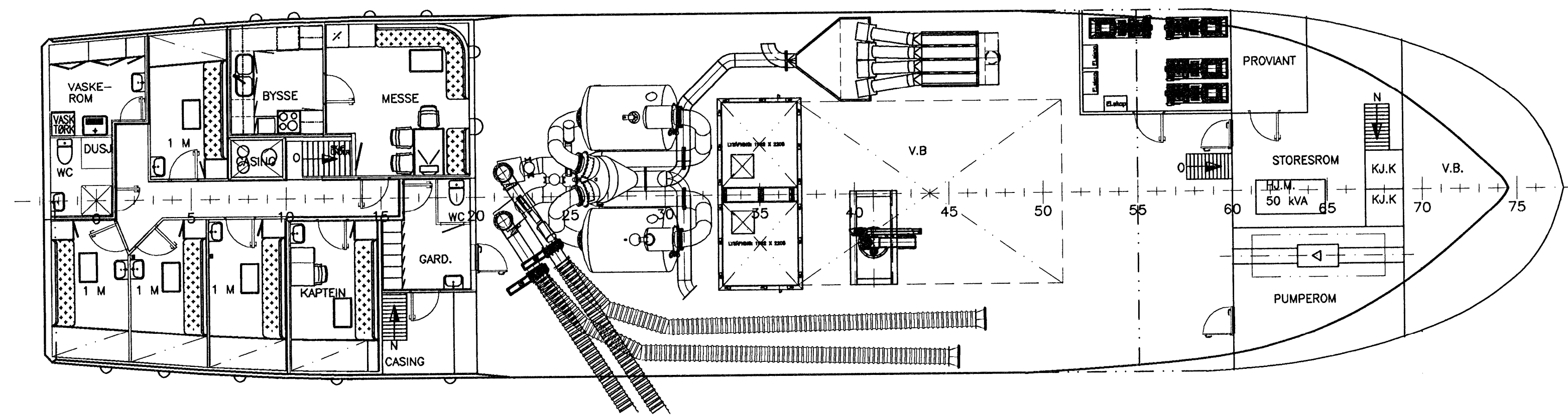
HOVEDDEKK
