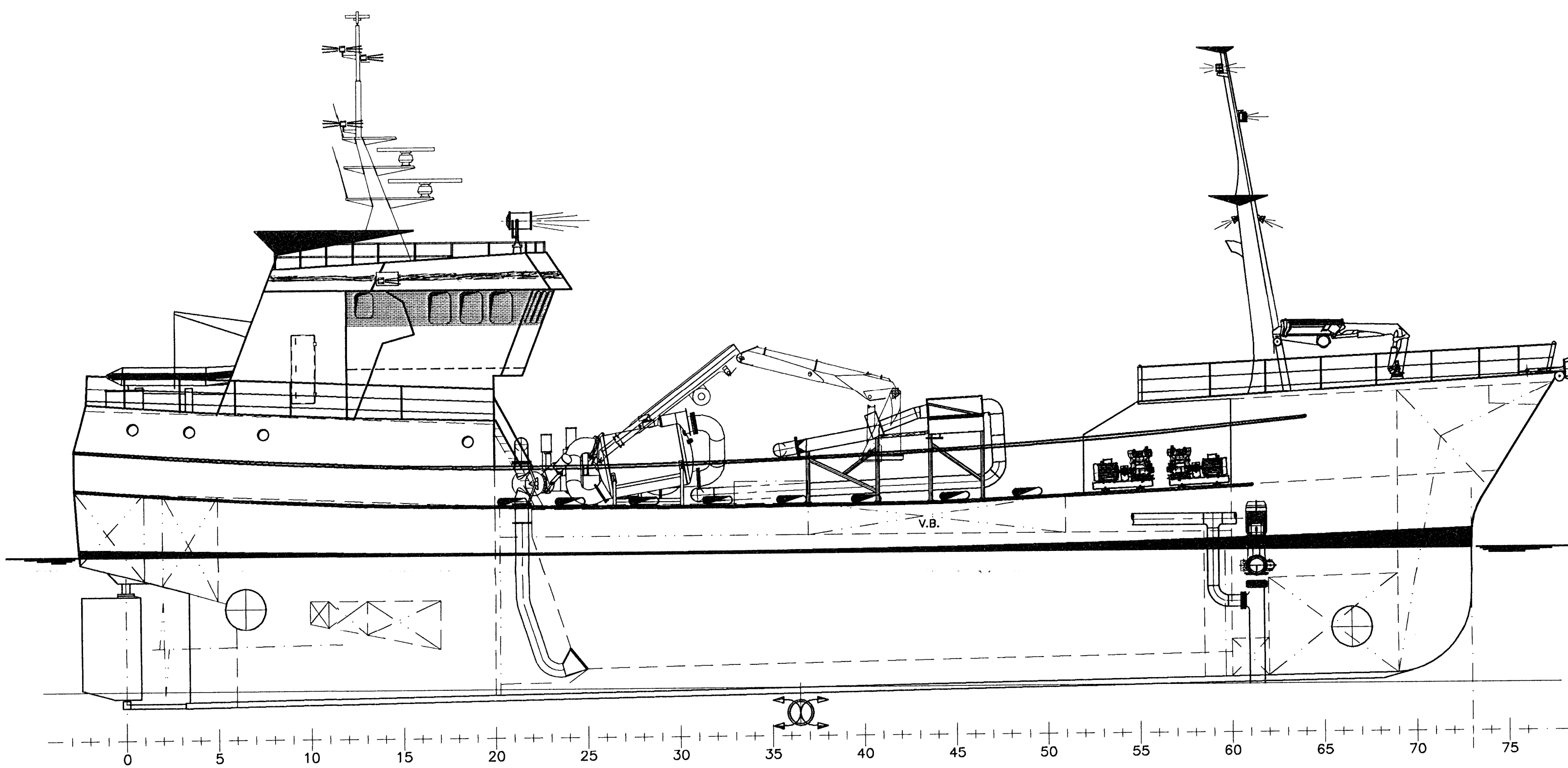
PROFIL
