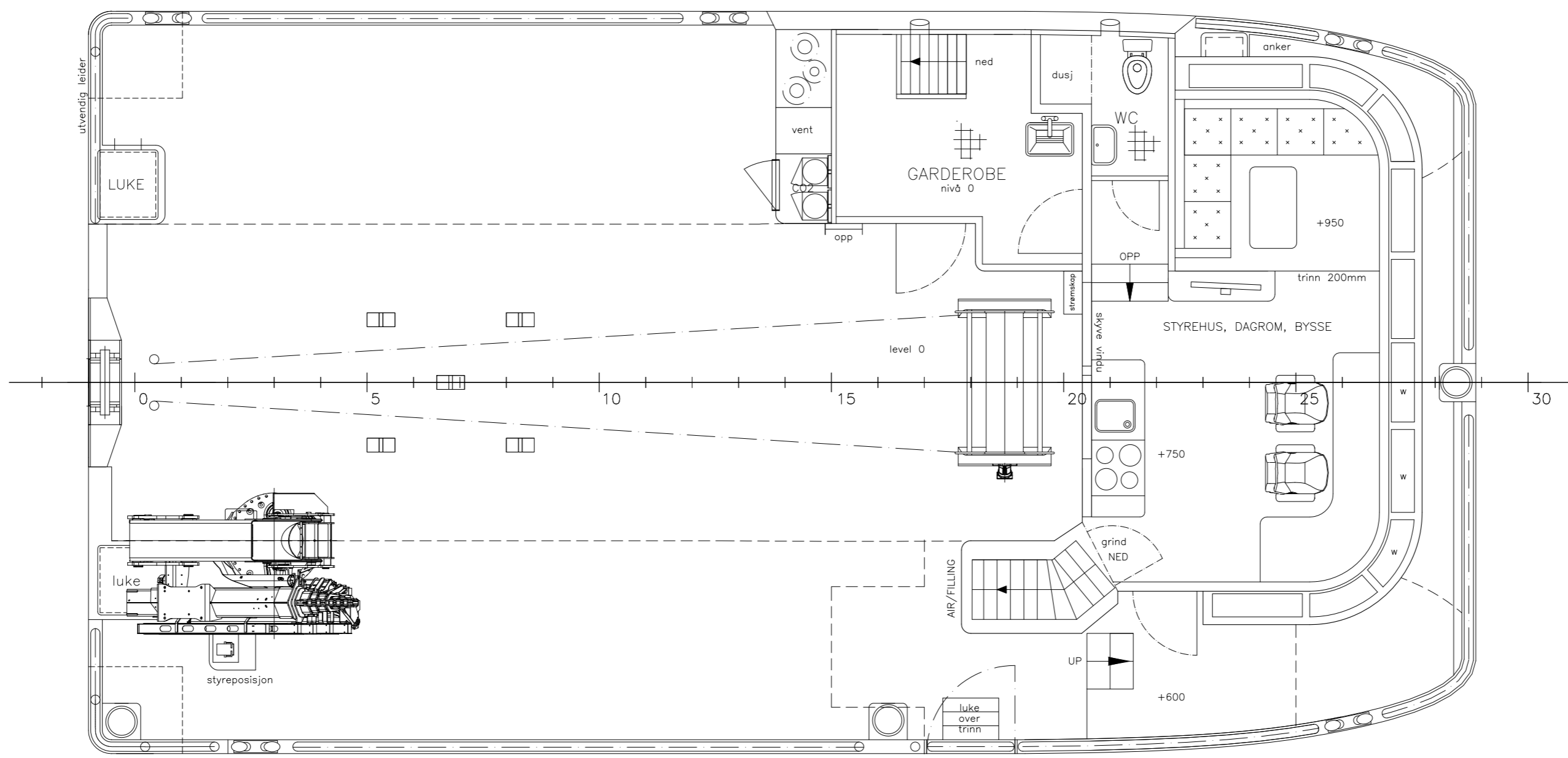
HOVEDDEKK
