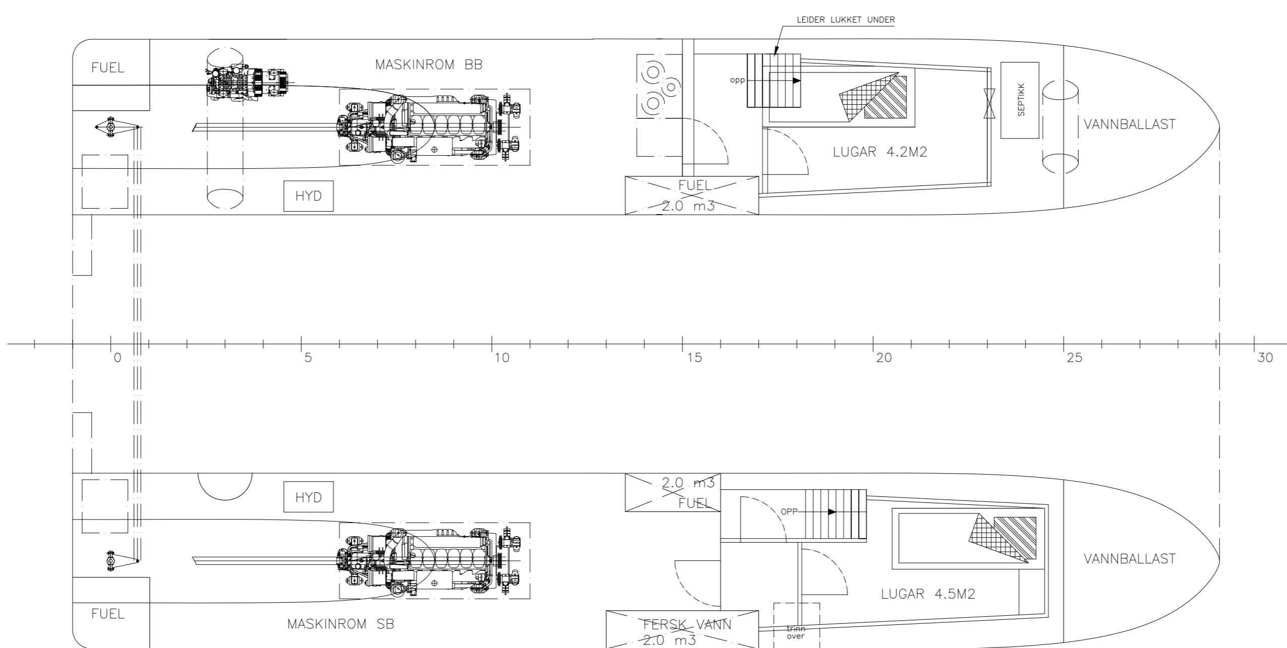
UNDER HOVEDDEKK
